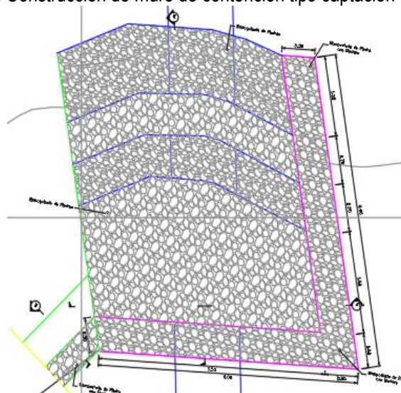
Figura 04. Construcción de muro de contención tipo captación en quebrada
